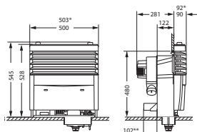
Monteringsmått S 3004
