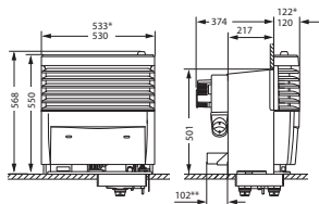
Monteringsmått S 5004
